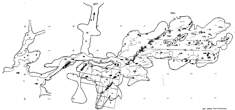
Περιστερία, Σπήλαιο Ευριπίδη. Κάτοψη των χώρων. Peristeria, Cave of Euripides. Plan.
