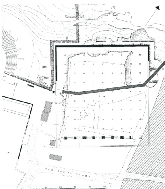
Εικ. 1. Κάτοψη (συμπληρωμένη) του Ωδείου του Περικλή στη νότια κλιτύ της Ακρόπολης των Αθηνών, κατά Ι. Τραυλό, 1971.
