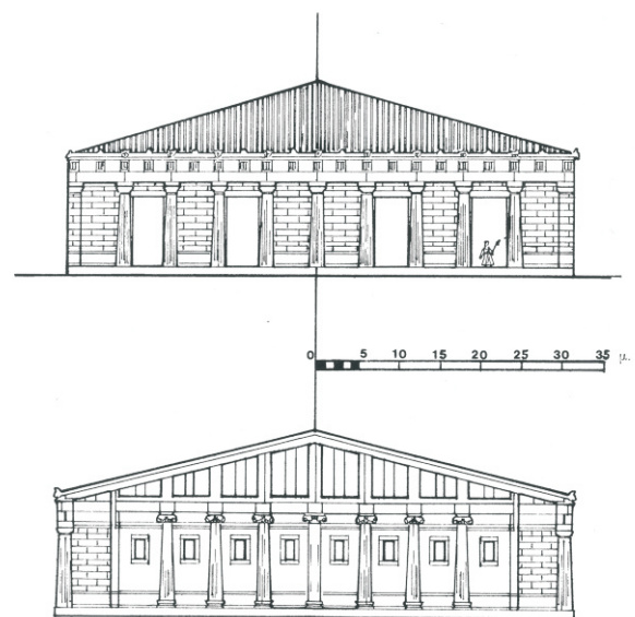
Εικ. 2. Αναπαράσταση του Ωδείου του Περικλή στα ανατολικά του Θεάτρου του Διονύσου, στη Ν. κλιτύ της Ακρόπολης των Αθηνών, κατά Α. Λ. Η. Ρομπκίν, 1979.
