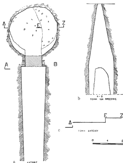
Εικ. 1. Σαλαμίς, Σελήνια (Λιμνιώνα). Σχέδια (κάτοψη και τομές) του Μυκηναϊκοῦ θαλαμοειδοῦς τάφου, καταχωσμένου σήμερα (κατὰ Α. Ἀνδρειωμένου 1961-1962).
