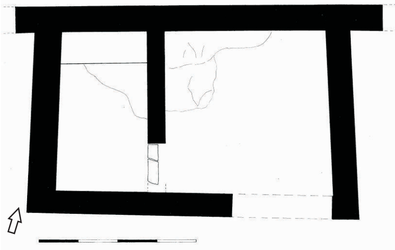
Εικ. 1. Κανάκια, Μυκηναϊκή ακρόπολη. Κάτοψη Προμαχώνα Ι (αποτύπωση: Χρ. Μαραμπέα, 2014).
