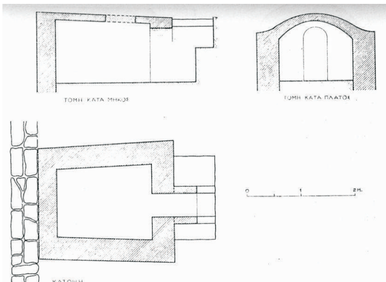
Σαλαμίς, Πυργιακόνι. Τομές και κάτοψη του χριστιανικού καμαρωτού τάφου που ερεύνησε ο Δημ. Πάλλας το 1987 (από Π.Α.Ε. 1987, Εικ. 1).
