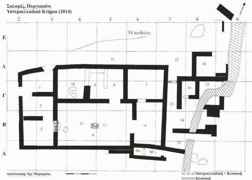
Εικ. 1. Πυργιακόνι. Κάτοψη του Υστεροελλαδικού επίσημου κτηρίου, 2014.
